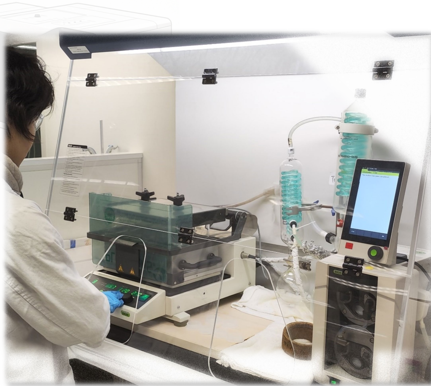
透過溶劑蒸發儀分析食品樣品中的總脂肪含量。
