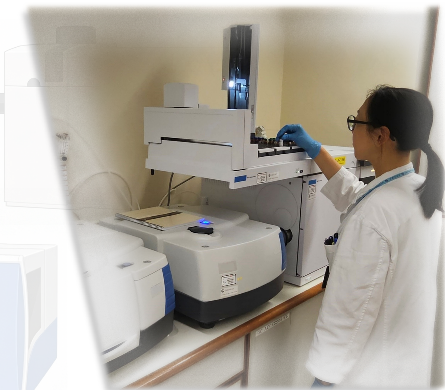
以氣相色譜傅里葉變換紅外線光譜儀系統分析耗蝕臭氧層物質 (ODS)。
