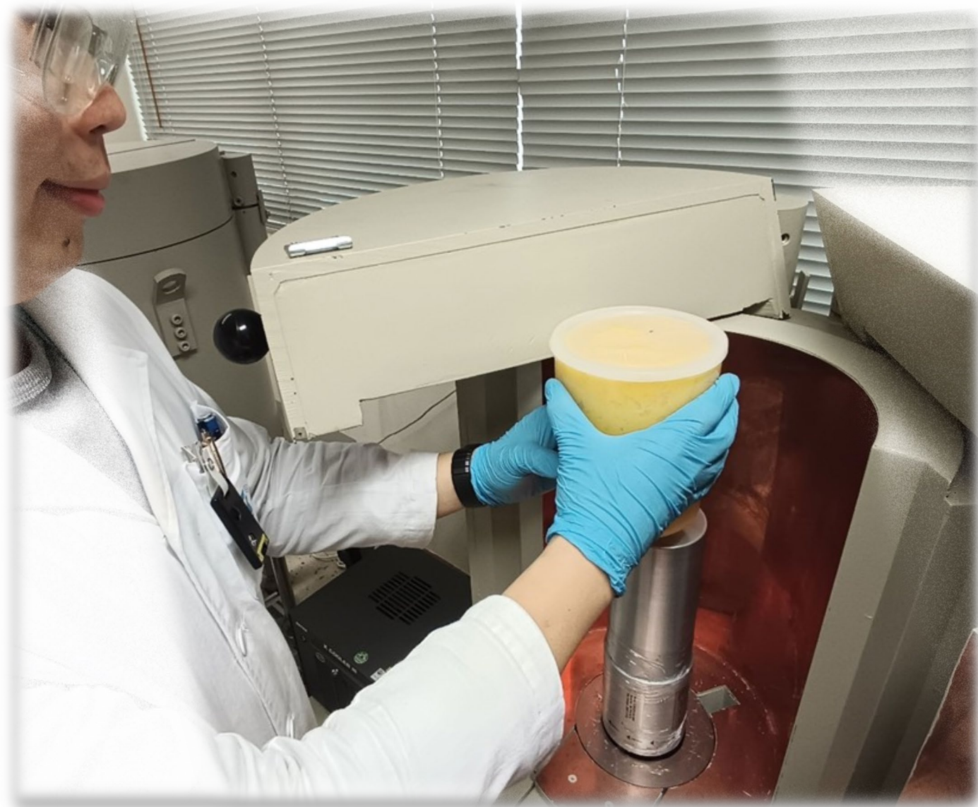
使用配備高純度銻探測器的伽瑪射線譜儀，分析進口食物樣本的放射性核素污染。
