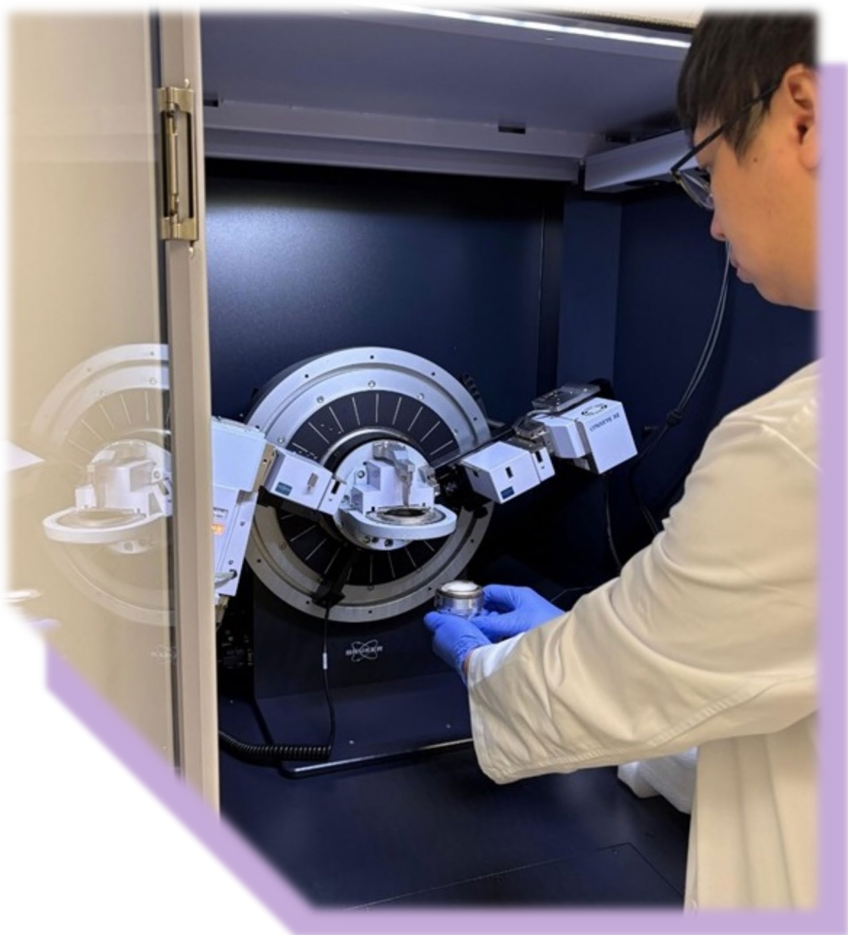
使用X射線衍射儀進行空氣中懸浮微粒分析。
